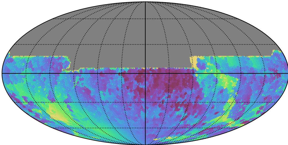
ddf_acor_sf30_lsf40_lsr20_v3.4_10yrs All sky y band: Min solarElong
