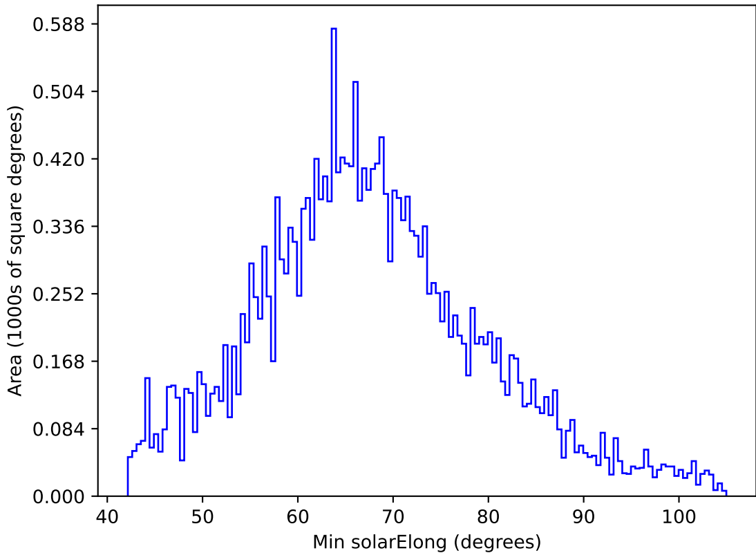
ddf_acor_sf30_lsf40_lsr20_v3.4_10yrs All sky y band: Min solarElong
