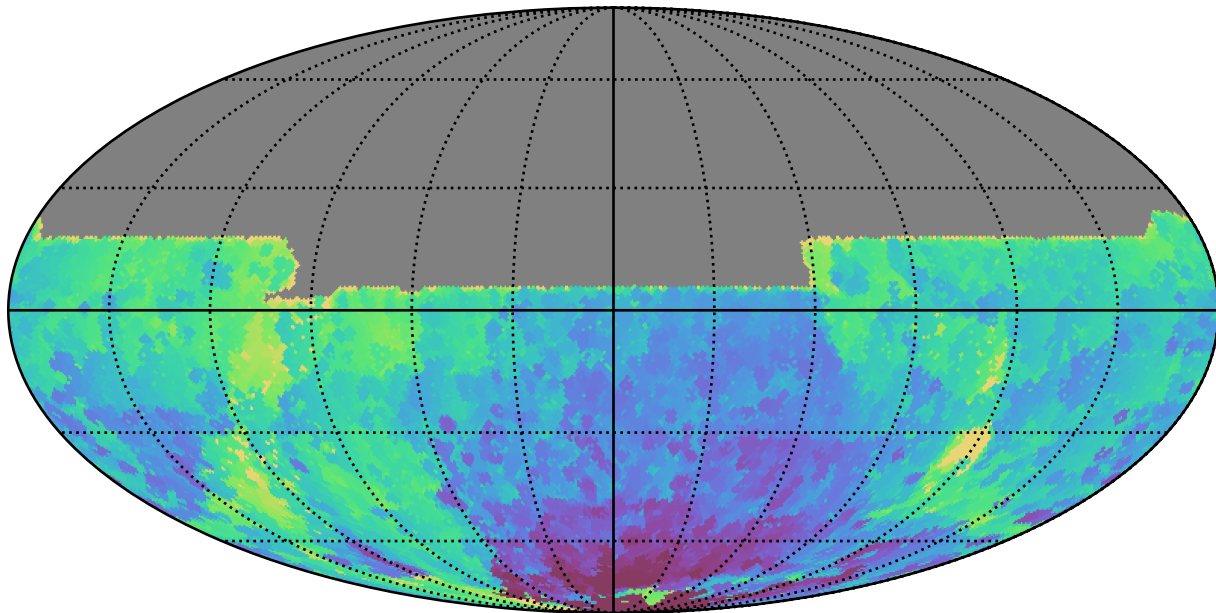
ddf_acor_sf30_lsf40_lsr20_v3.4_10yrs All sky y band: Min HA
