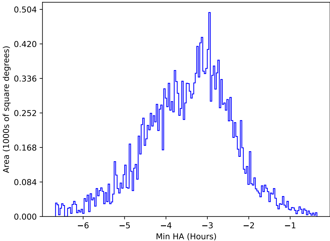
ddf_acor_sf30_lsf40_lsr20_v3.4_10yrs All sky y band: Min HA
