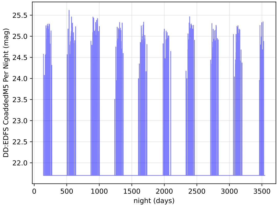
ddf_acor_sf30_lsf40_lsr20_v3.4_10yrs z band: DD:EDFS CoaddedM5 Per Night
