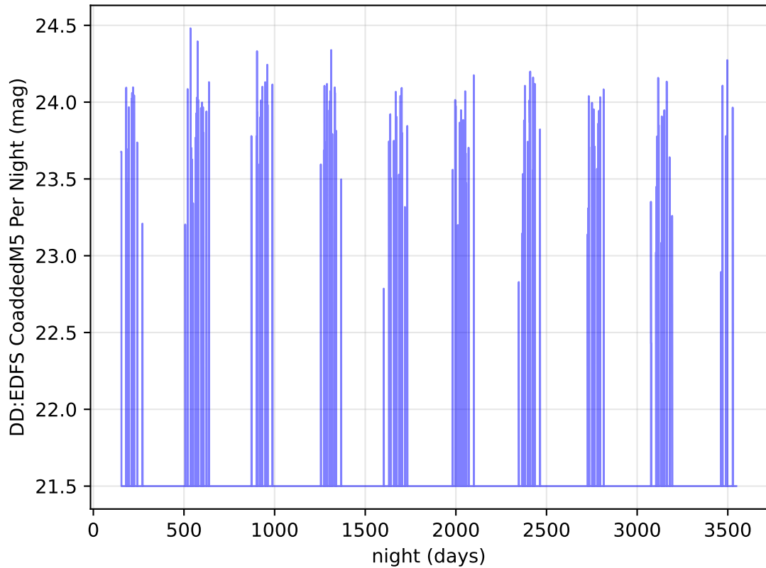
ddf_acor_sf30_lsf40_lsr20_v3.4_10yrs y band: DD:EDFS CoaddedM5 Per Night
