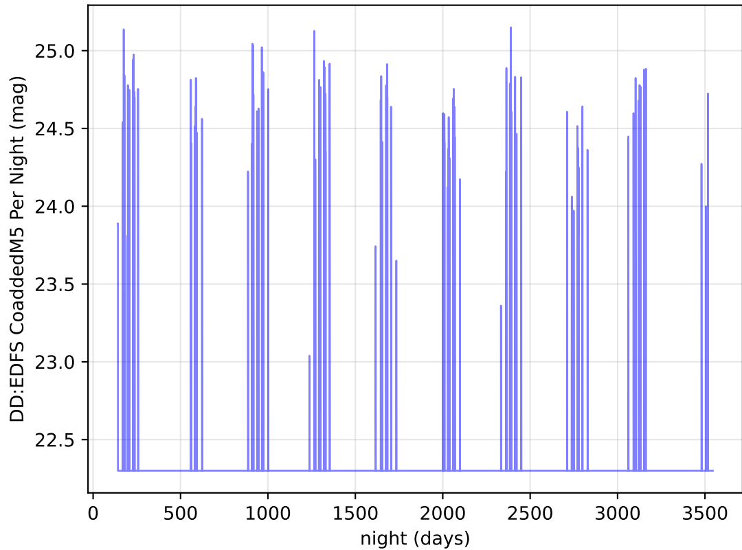
ddf_acor_sf30_lsf40_lsr20_v3.4_10yrs u band: DD:EDFS CoaddedM5 Per Night
