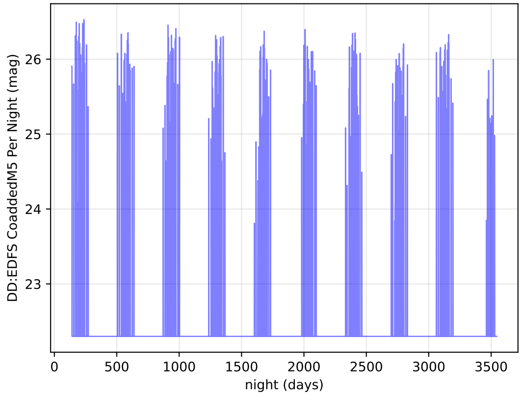
ddf_acor_sf30_lsf40_lsr20_v3.4_10yrs g band: DD:EDFS CoaddedM5 Per Night
