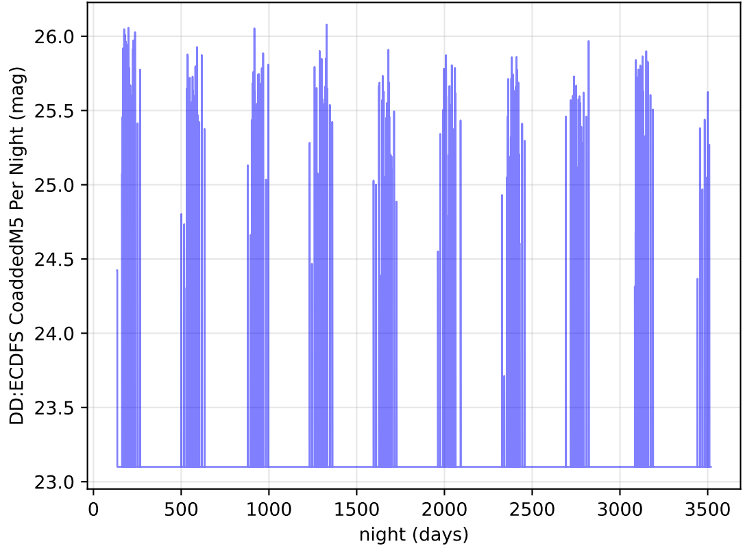
ddf_acor_sf30_lsf40_lsr20_v3.4_10yrs i band: DD:ECDFS CoaddedM5 Per Night
