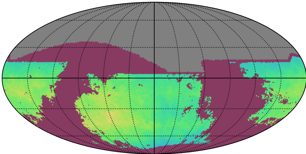
ddf_acor_sf30_lsf40_lsr10_v3.4_10yrs i: NgalScale
