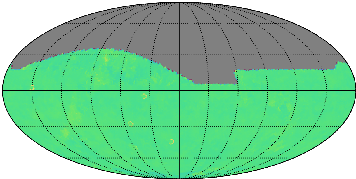
ddf_acor_sf30_lsf40_lsr10_v3.4_10yrs z: Kuiper rotTelPos
