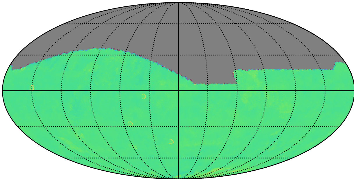
ddf_acor_sf30_lsf40_lsr10_v3.4_10yrs r: Kuiper rotTelPos
