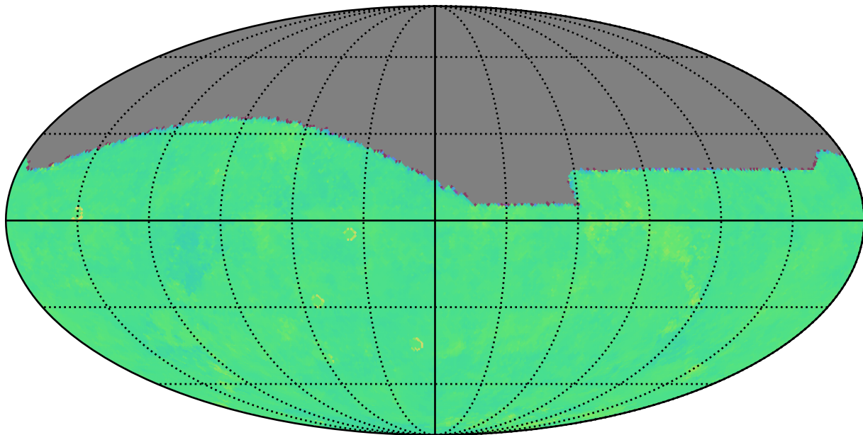
ddf_acor_sf30_lsf40_lsr10_v3.4_10yrs g: Kuiper rotTelPos
