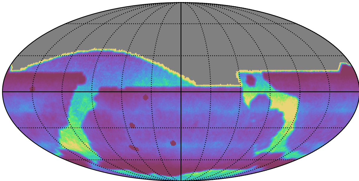
ddf_acor_sf30_lsf40_lsr10_v3.4_10yrs : DCRprecision
