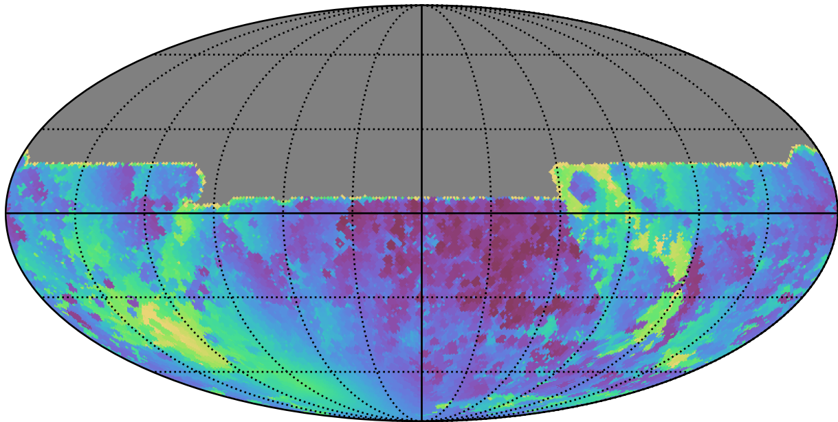
ddf_acor_sf30_lsf40_lsr10_v3.4_10yrs All sky y band: Min solarElong
