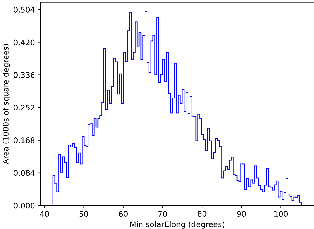
ddf_acor_sf30_lsf40_lsr10_v3.4_10yrs All sky y band: Min solarElong
