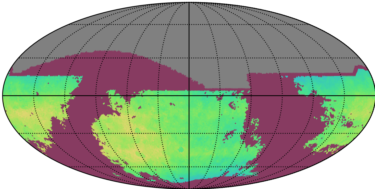
ddf_acor_sf25_lsf40_lsr50_v3.4_10yrs i: NgalScale
