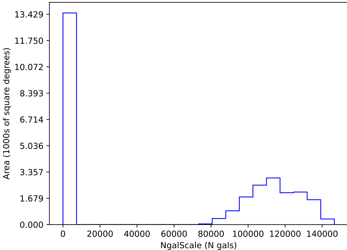
ddf_acor_sf25_lsf40_lsr50_v3.4_10yrs i: NgalScale
