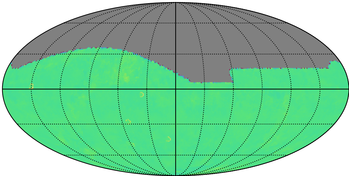
ddf_acor_sf25_lsf40_lsr50_v3.4_10yrs i: Kuiper rotTelPos
