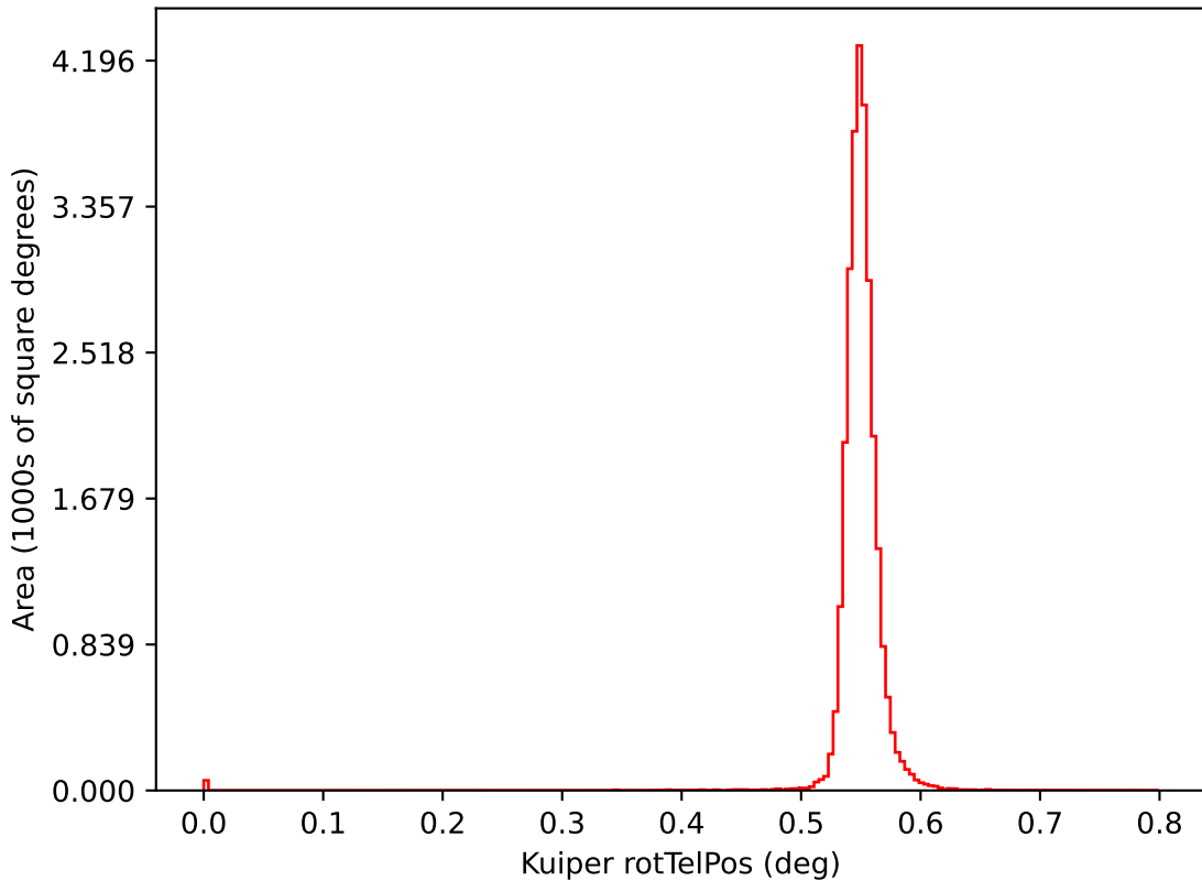
ddf_acor_sf25_lsf40_lsr50_v3.4_10yrs i: Kuiper rotTelPos
