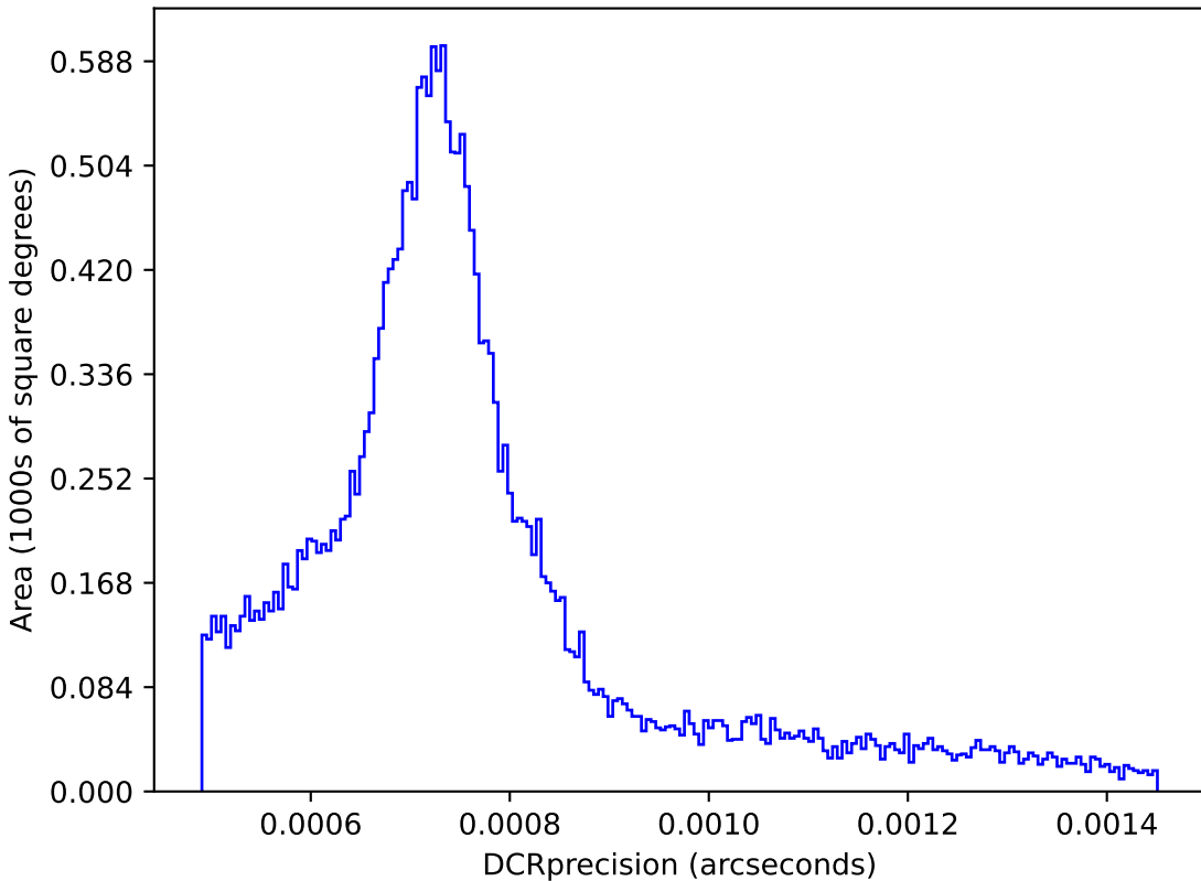
ddf_acor_sf25_lsf40_lsr50_v3.4_10yrs : DCRprecision
