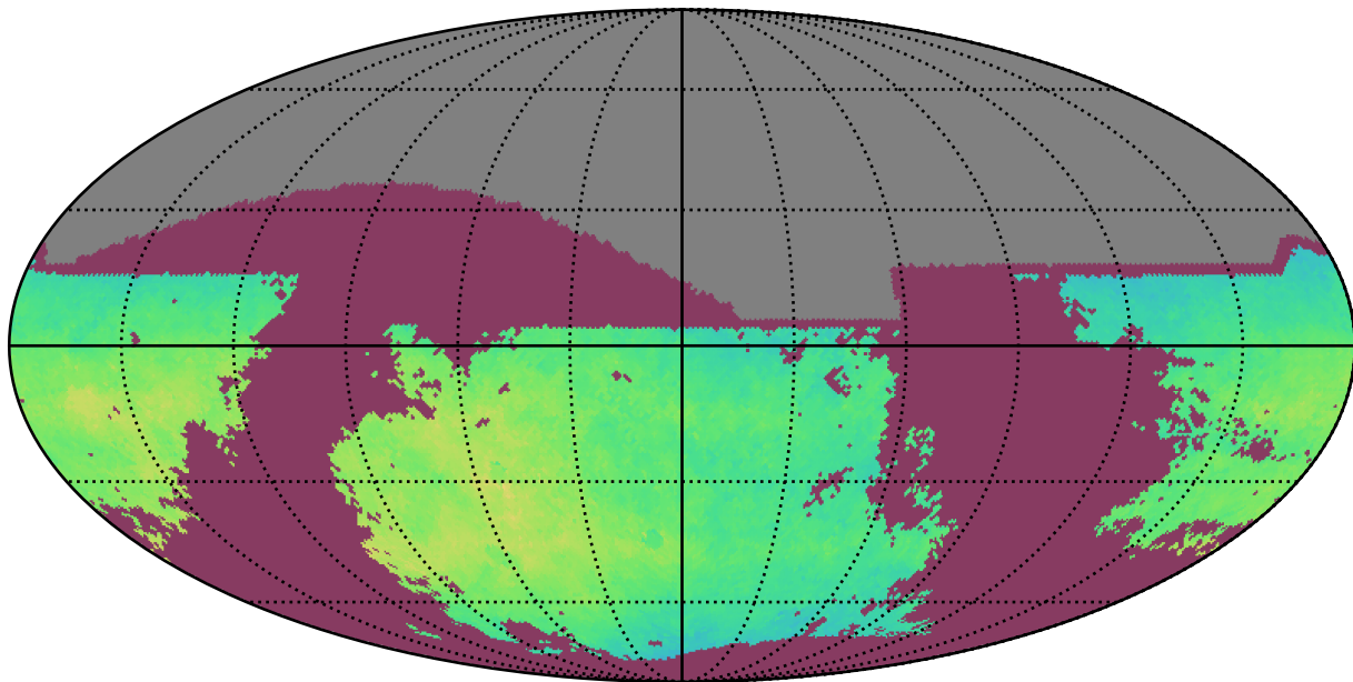
ddf_acor_sf25_lsf40_lsr20_v3.4_10yrs i: NgalScale
