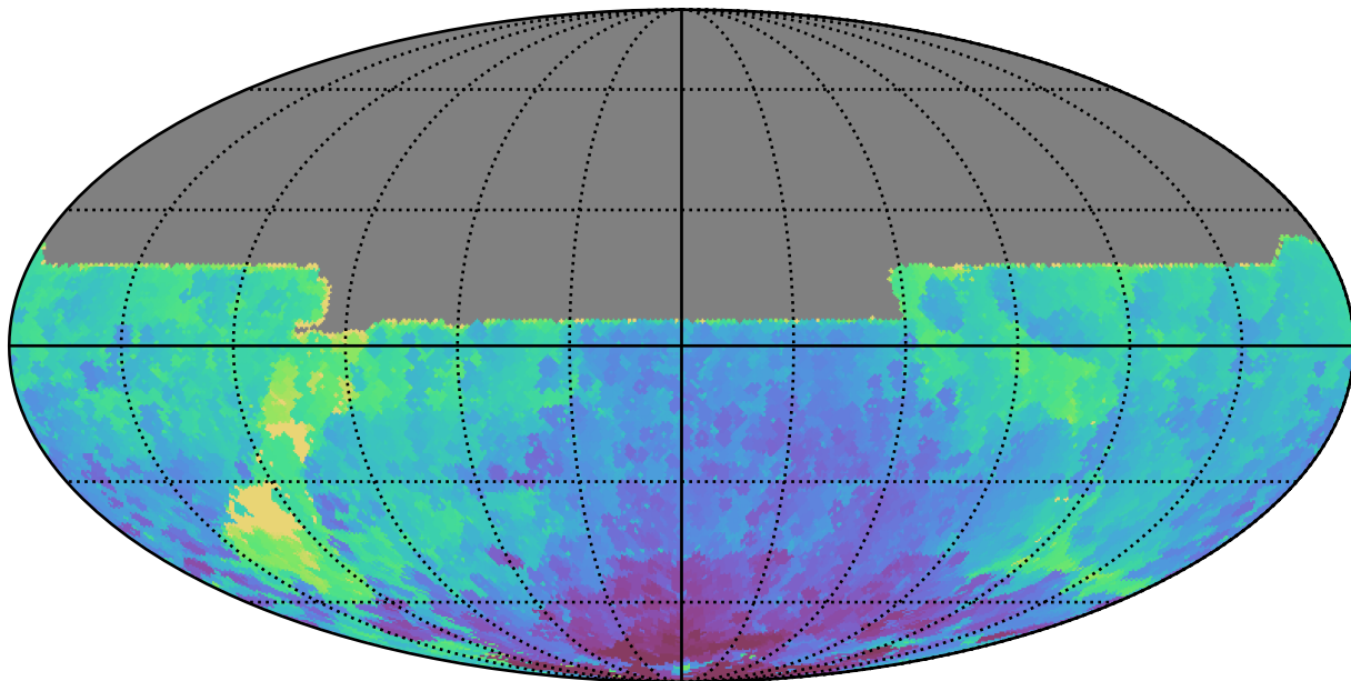
ddf_acor_sf25_lsf40_lsr20_v3.4_10yrs All sky y band: Min HA
