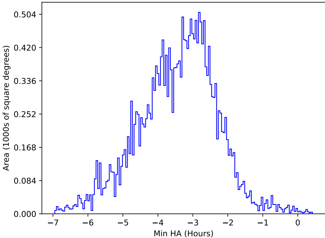
ddf_acor_sf25_lsf40_lsr20_v3.4_10yrs All sky y band: Min HA
