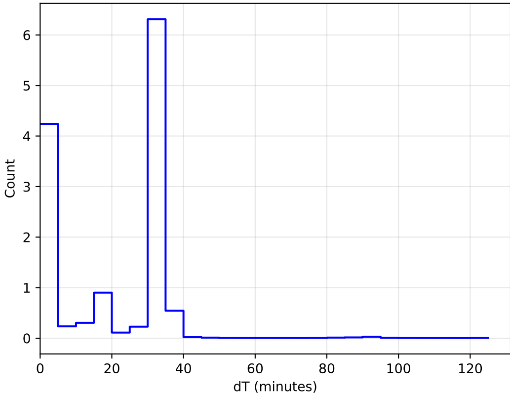
ddf_acor_sf25_lsf40_lsr20_v3.4_10yrs All sky: DeltaT Histogram 1e6
