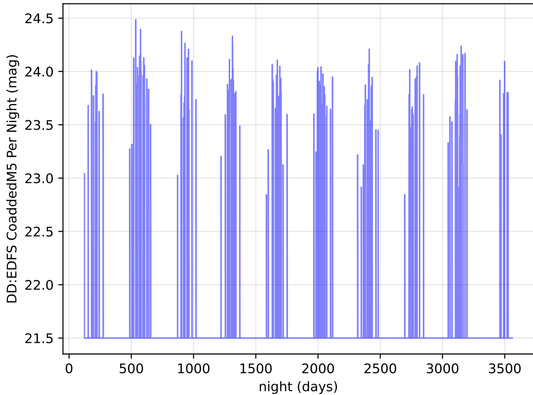
ddf_acor_sf25_lsf40_lsr20_v3.4_10yrs y band: DD:EDFS CoaddedM5 Per Night
