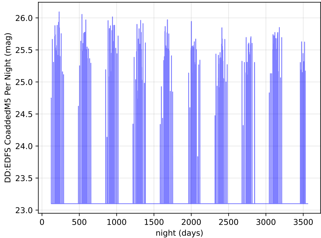
ddf_acor_sf25_Isf40_Isr20_v3.4_10yrs i band: DD:EDFS CoaddedM5 Per Night
