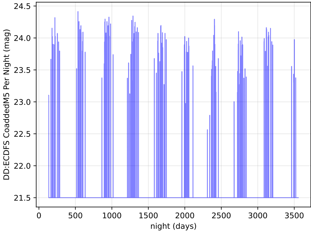
ddf_acor_sf25_lsf40_lsr20_v3.4_10yrs y band: DD:ECDFS CoaddedM5 Per Night
