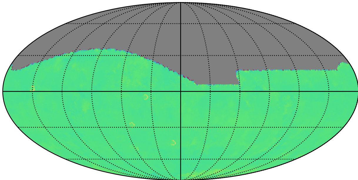
ddf_acor_sf25_lsf40_lsr10_v3.4_10yrs r: Kuiper rotTelPos
