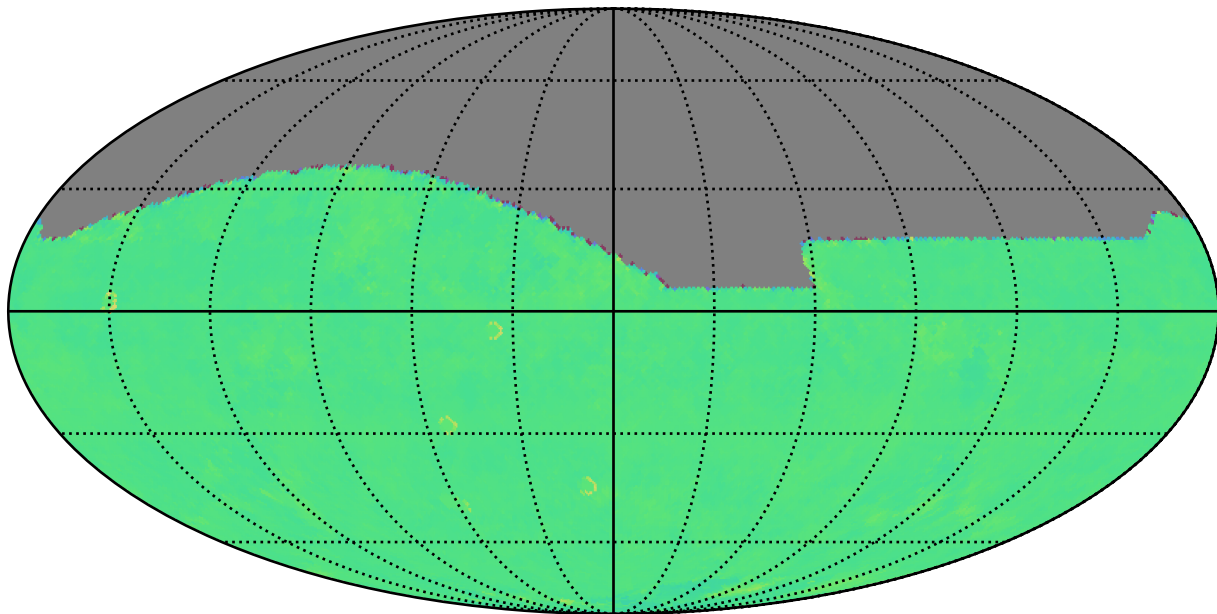
ddf_acor_sf25_lsf40_lsr10_v3.4_10yrs i: Kuiper rotTelPos
