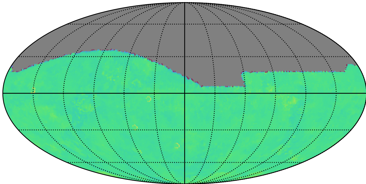
ddf_acor_sf25_lsf40_lsr10_v3.4_10yrs g: Kuiper rotTelPos
