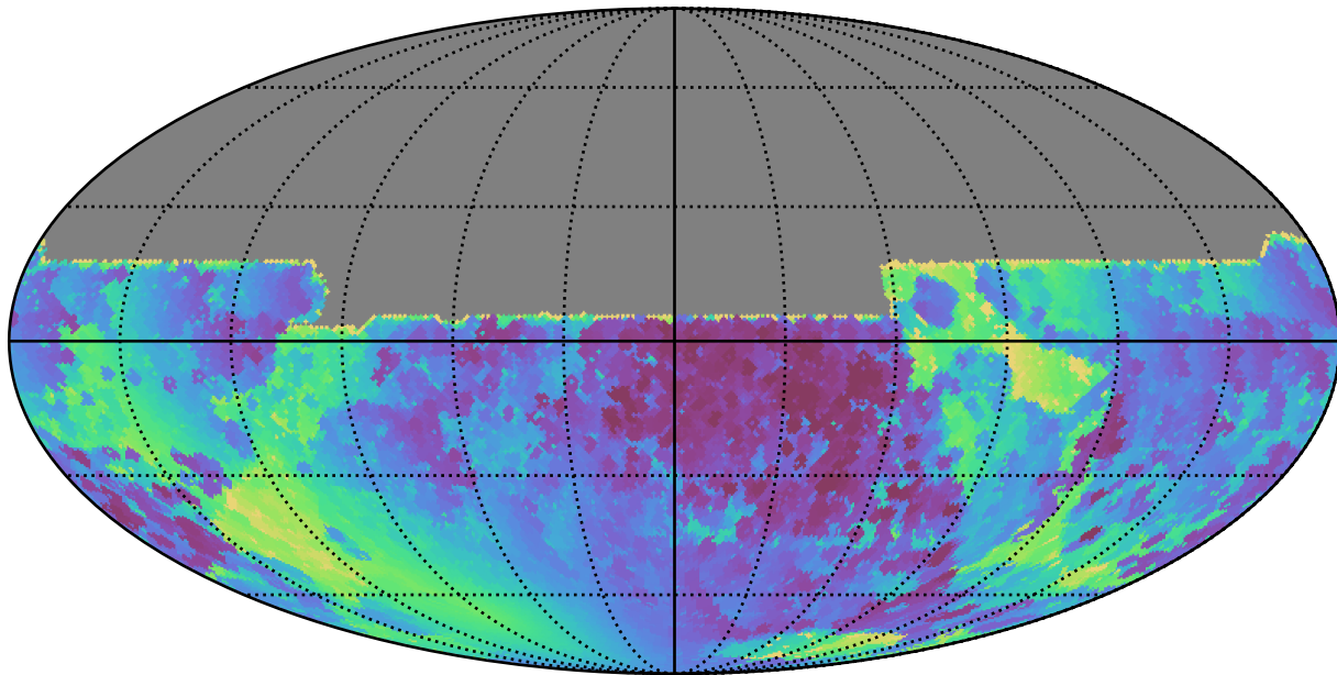
ddf_acor_sf25_lsf40_lsr10_v3.4_10yrs All sky y band: Min solarElong
