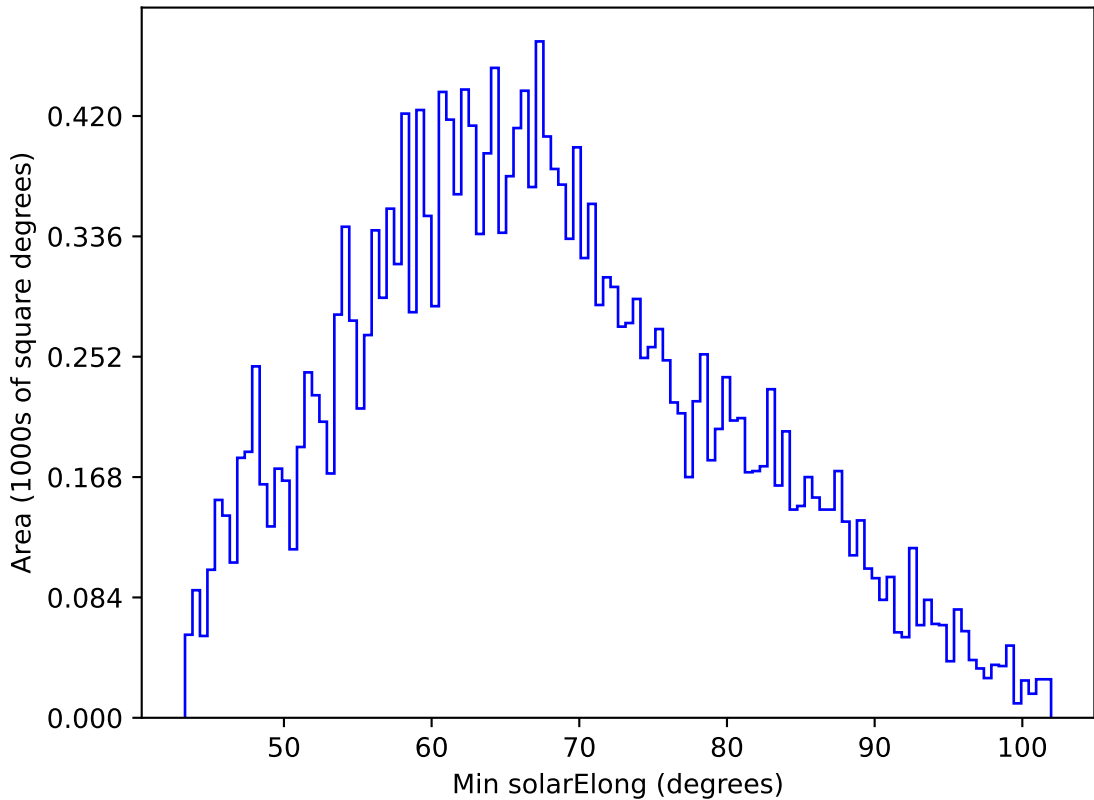
ddf_acor_sf25_lsf40_lsr10_v3.4_10yrs All sky y band: Min solarElong
