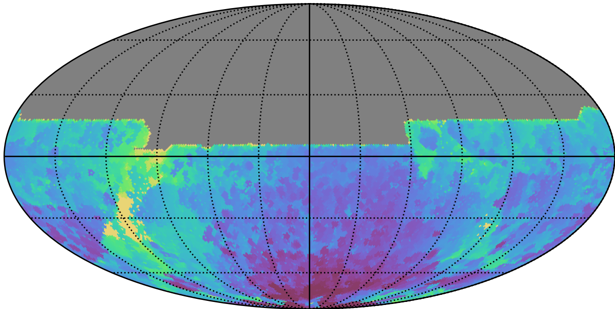
ddf_acor_sf25_lsf40_lsr10_v3.4_10yrs All sky y band: Min HA
