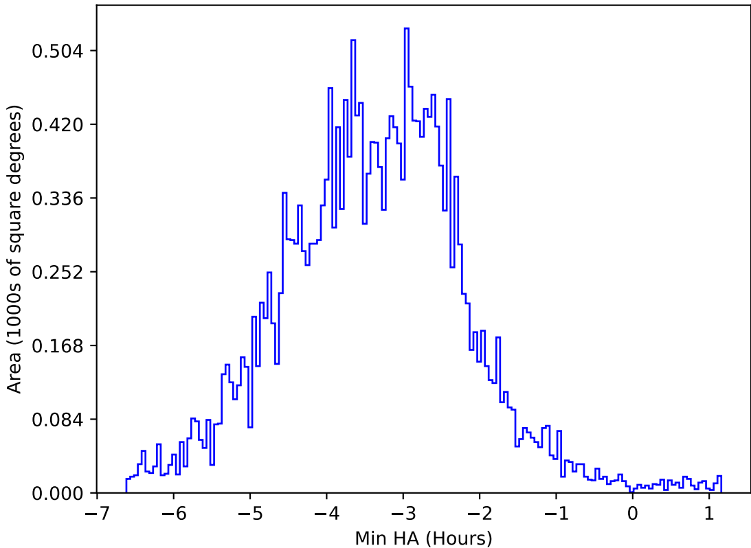
ddf_acor_sf25_lsf40_lsr10_v3.4_10yrs All sky y band: Min HA
