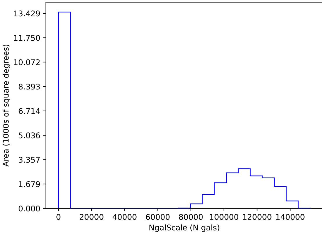
ddf_acor_sf25_lsf30_lsr50_v3.4_10yrs i: NgalScale
