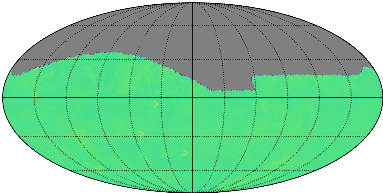
ddf_acor_sf25_lsf30_lsr50_v3.4_10yrs i: Kuiper rotTelPos
