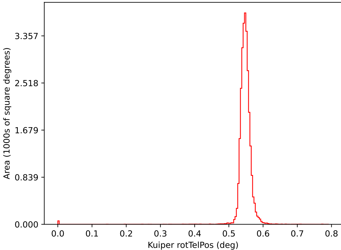
ddf_acor_sf25_lsf30_lsr50_v3.4_10yrs i: Kuiper rotTelPos
