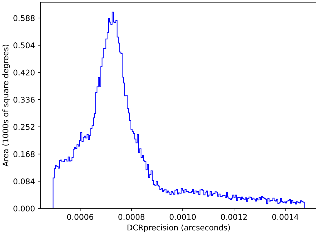
ddf_acor_sf25_lsf30_lsr50_v3.4_10yrs : DCRprecision
