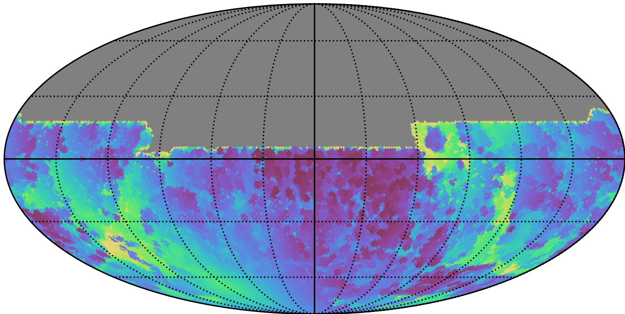
ddf_acor_sf25_lsf30_lsr50_v3.4_10yrs All sky y band: Min solarElong
