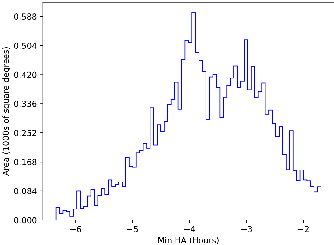
ddf_acor_sf25_lsf30_lsr50_v3.4_10yrs WFD y band: Min HA
