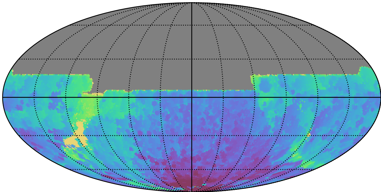
ddf_acor_sf25_lsf30_lsr50_v3.4_10yrs All sky y band: Min HA
