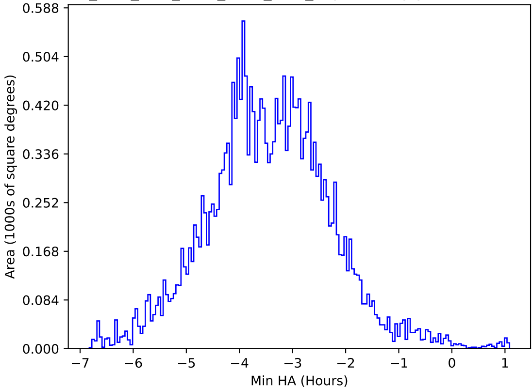
ddf_acor_sf25_lsf30_lsr50_v3.4_10yrs All sky y band: Min HA
