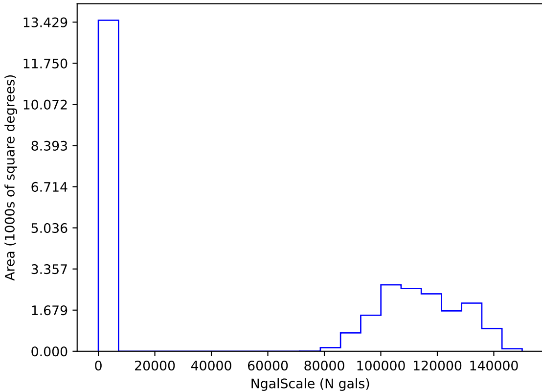
ddf_acor_sf25_lsf30_lsr20_v3.4_10yrs i: NgalScale
