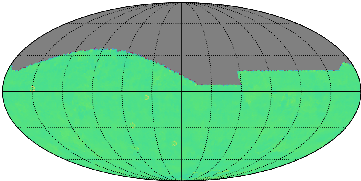
ddf_acor_sf25_lsf30_lsr20_v3.4_10yrs i: Kuiper rotTelPos
