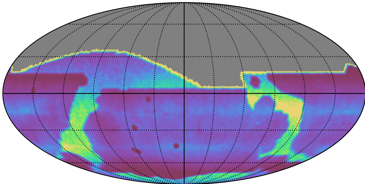
ddf_acor_sf25_lsf30_lsr20_v3.4_10yrs : DCRprecision
