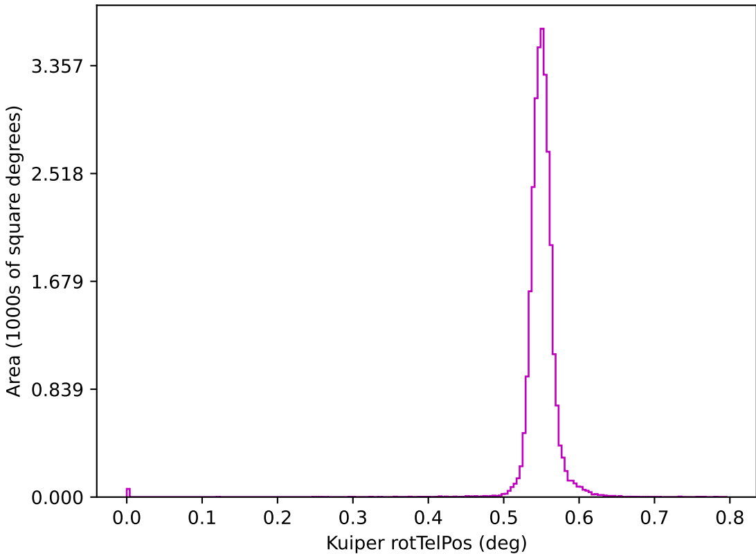
ddf_acor_sf25_lsf30_lsr10_v3.4_10yrs z: Kuiper rotTelPos
