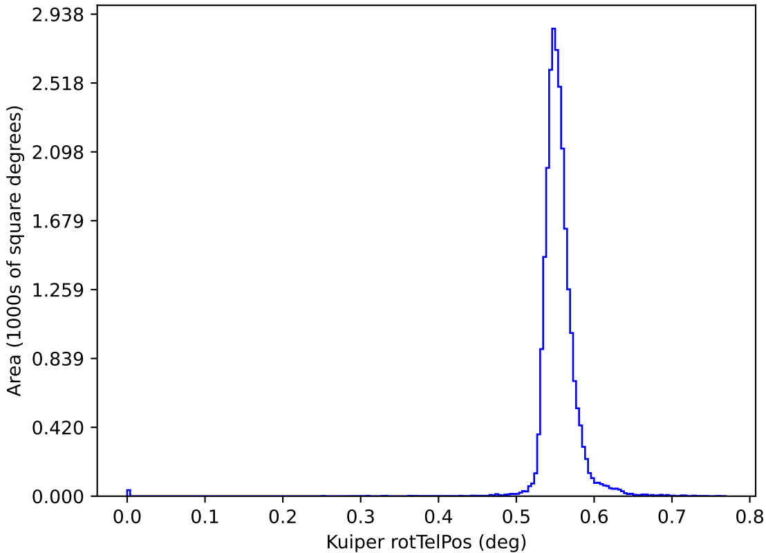
ddf_acor_sf25_lsf30_lsr10_v3.4_10yrs y: Kuiper rotTelPos
