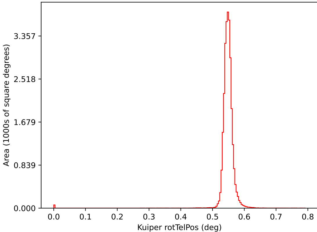
ddf_acor_sf25_lsf30_lsr10_v3.4_10yrs i: Kuiper rotTelPos
