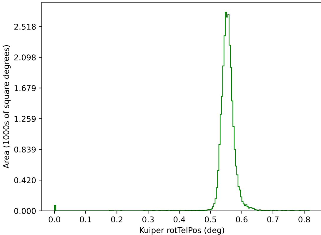
ddf_acor_sf25_ls30_lsr10_v3.4_10yrs g: Kuiper rotTelPos
